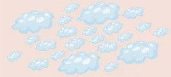
ALTOCÚMULUS
